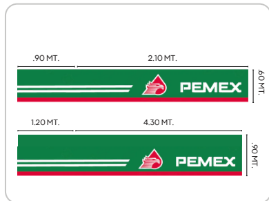
Lona Caja Muerto Trad Tipo A y B
